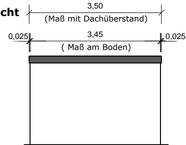
Rückansicht
