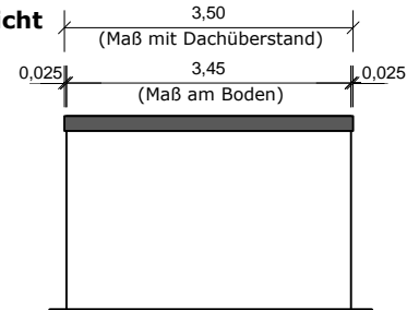
Rückansicht
